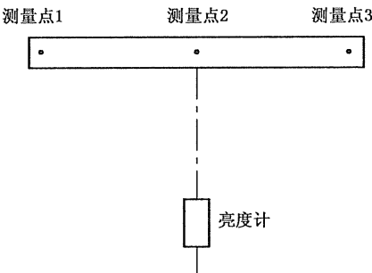
图 A.1 亮度测量图示
